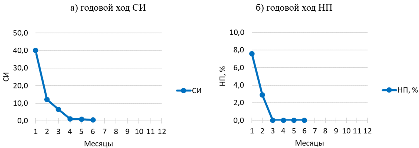
Рис. 18 — Годовой ход СИ и НП
